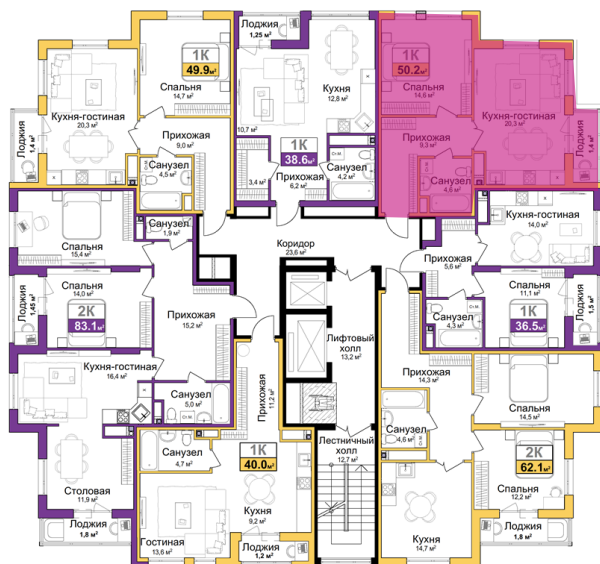
План этажа
