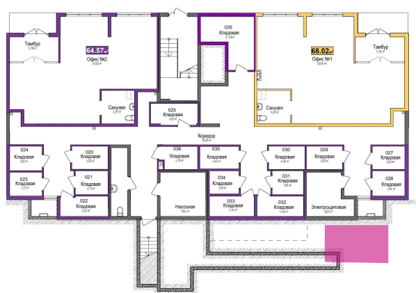
План этажа
