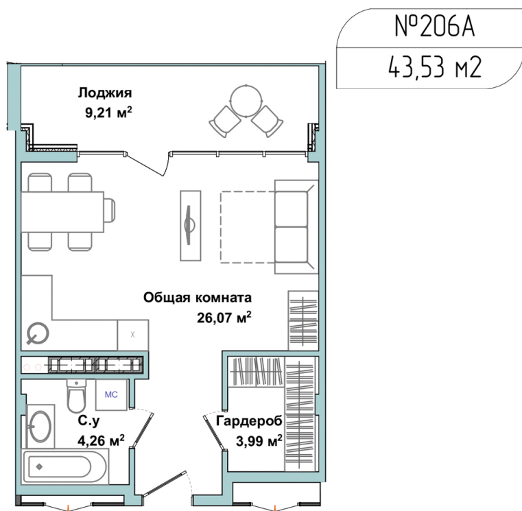
Планировка
