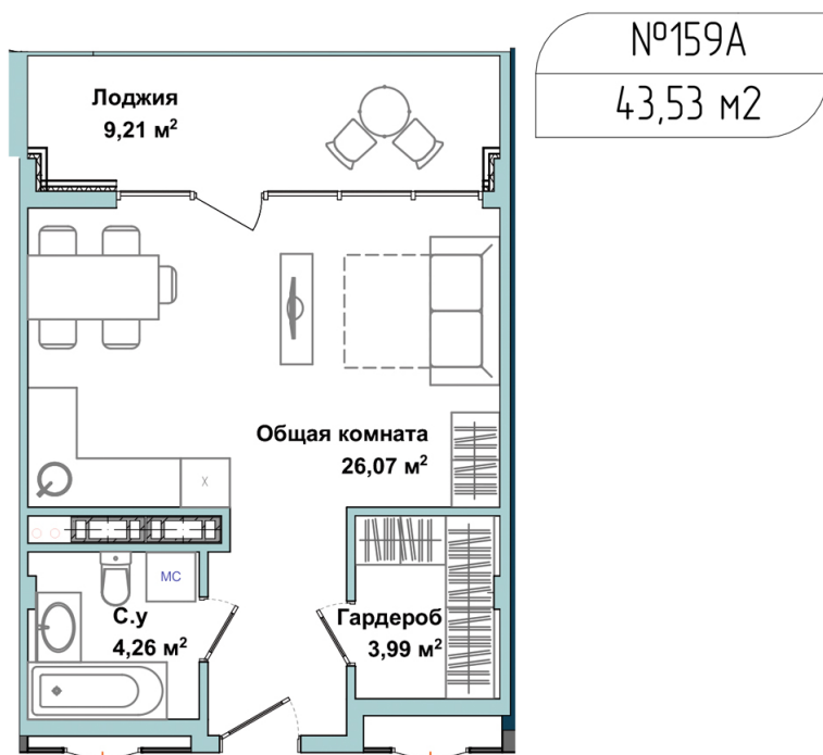
План этажа
