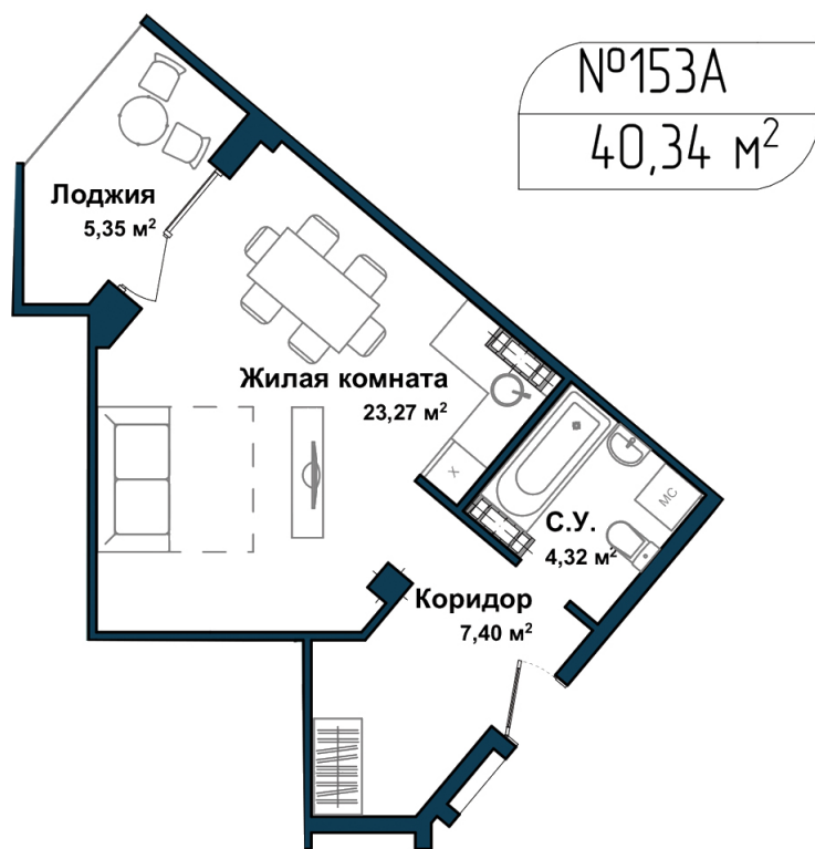
План этажа
