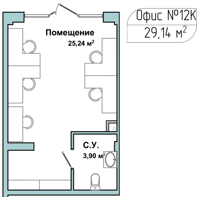
План этажа
