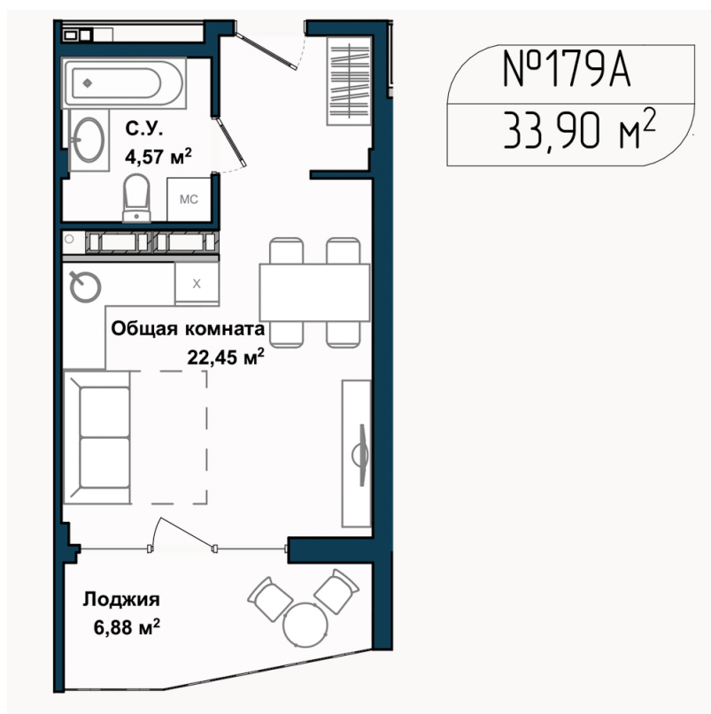
Планировка
