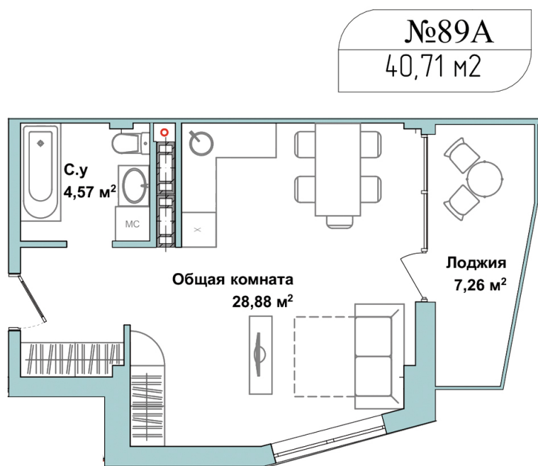
План этажа
