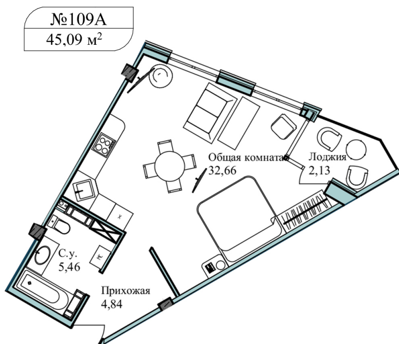
План этажа
