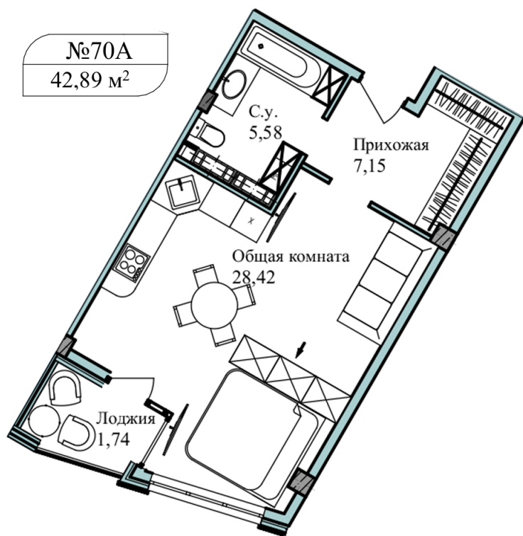
План этажа
