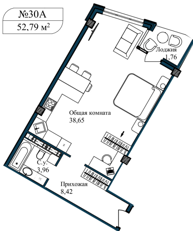
Планировка
