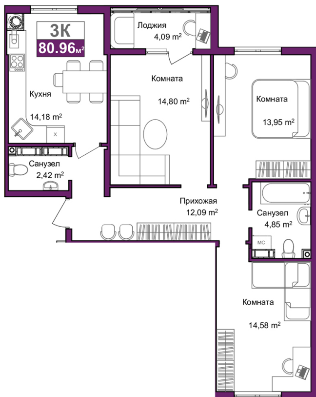
Планировка
