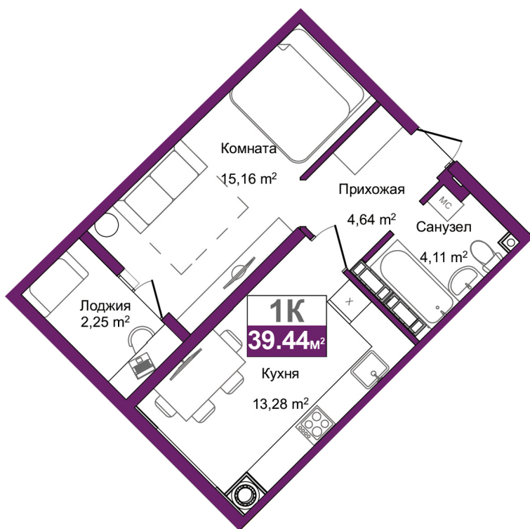
Планировка
