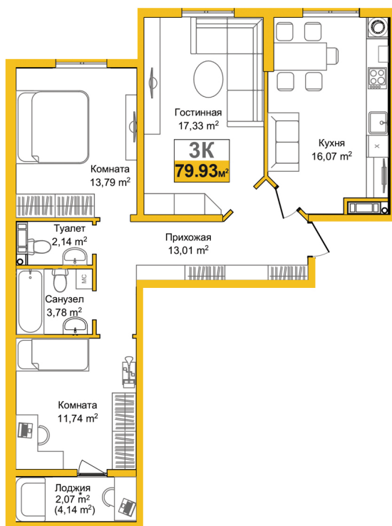
Планировка
