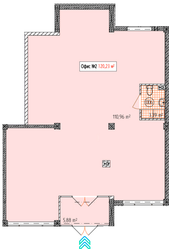
Планировка
